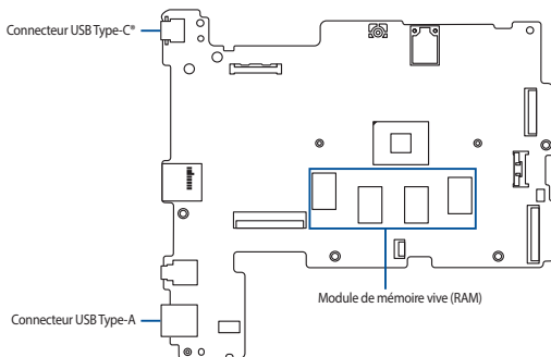
Carte mère avec ses ports et connecteurs
