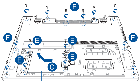
Zásuvka pre pevnú diskovú jednotku
