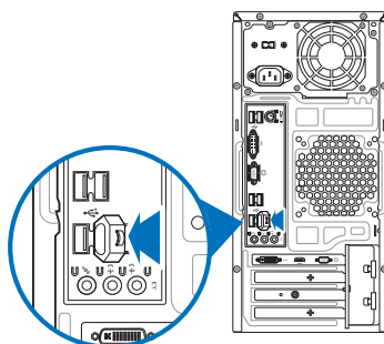
Panneau arrière
