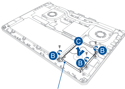
відсік для жорсткого диска
