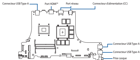
Carte mère avec ses ports et connecteurs
