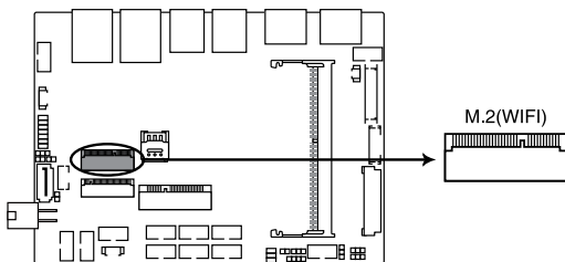
M.2(WIFI) slot
