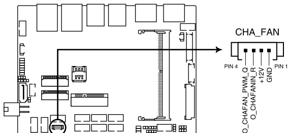
FAN connector
