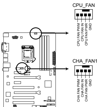
B85-A Fan connectors
