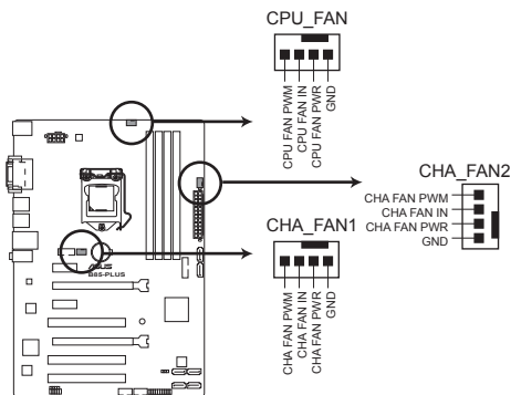
Connecteurs de ventilation de la B85-PLUS
