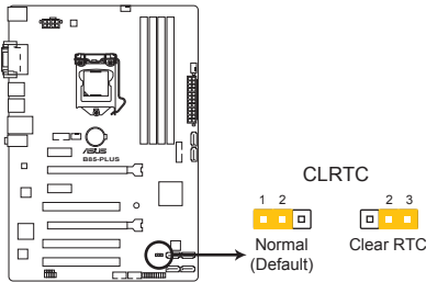
Jumper d'effacement de la mémoire CMOS de la B85-PLUS
