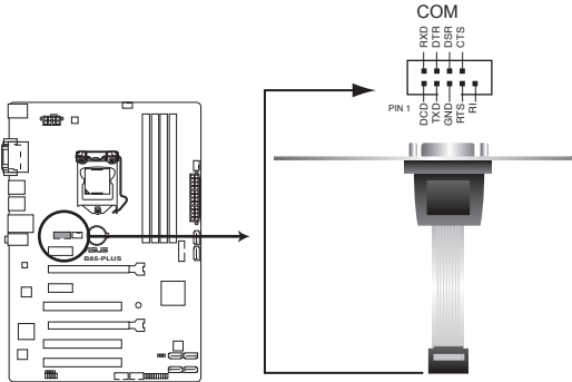
Connecteur pour port COM de la B85-PLUS
