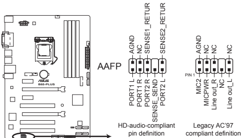
Connecteur audio pour panneau avant de la B85-PLUS
