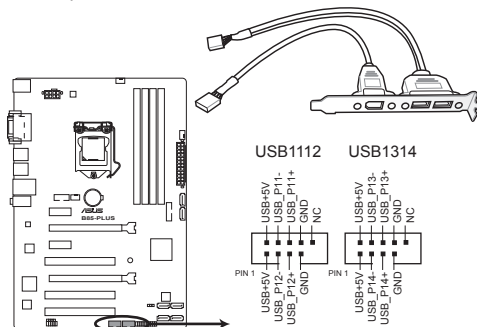
Connecteurs USB 2.0 de la B85-PLUS
