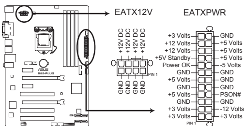
Connecteurs d'alimentation de la B85-PLUS
