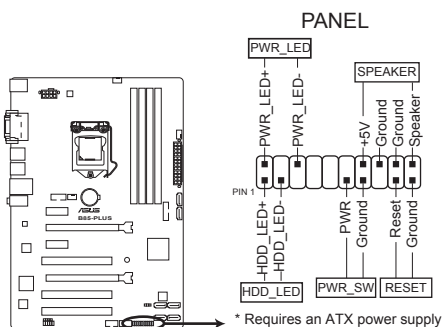
Connecteur panneau système de la B85-PLUS
