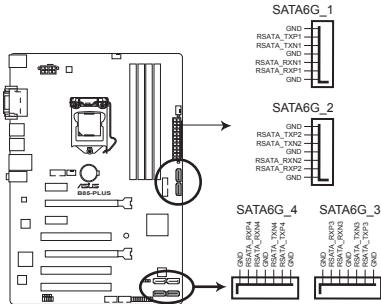
Connecteurs SATA 6.0Gbs de la B85-PLUS
