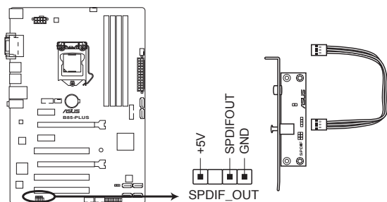
Connecteur audio numérique de la B85-PLUS
