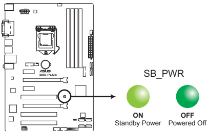
Voyant d'alimentation de la B85-PLUS
