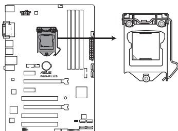
Interface de connexion LGA1150 de la B85-PLUS
