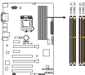
Interfaces de connexion pour modules mémoire DDR3 de la B85-PLUS
