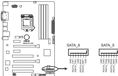
Connecteurs SATA 3.0Gbs de la B85-PLUS
