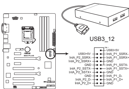
Connecteur USB 3.0 de la B85-PLUS
