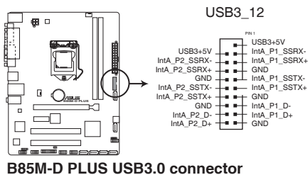
B85M-D PLUS USB3.0 connector
