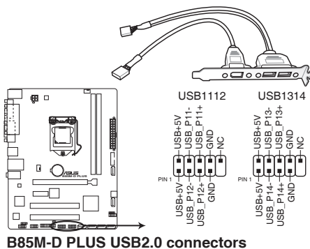
B85M-D PLUS USB2.0 connectors
