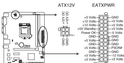
Connecteurs d'alimentation de la B85M-K
