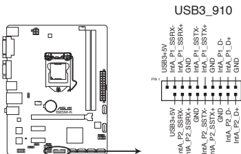
Connecteur USB 3.0 de la B85M-K
