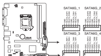
Connecteurs SATA 6.0Gbs de la B85M-K
