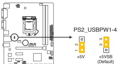
Jumper de mise en route via clavier et USB de la B85M-K
