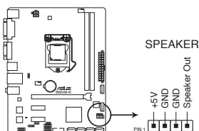
Connecteur pour haut-parleur d'alerte système de la B85M-K
