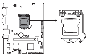
Interface de connexion LGA1150 de la B85M-K
