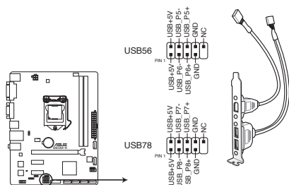
Connecteurs USB 2.0 de la B85M-K
