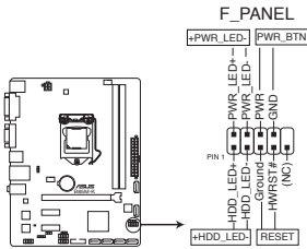
Connecteur panneau système de la B85M-K
