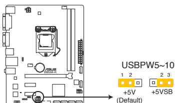
Jumper de mise en route via USB de la B85M-K
