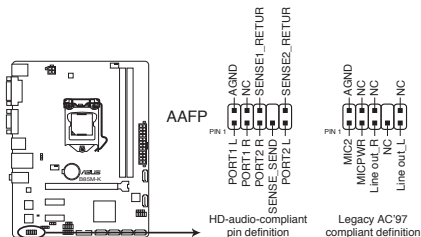
Connecteur audio pour panneau avant de la B85M-K
