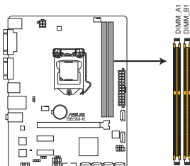
Interfaces de connexion pour modules mémoire DDR3 de la B85M-K
