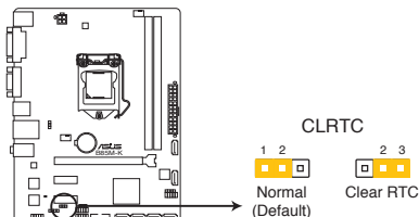
Jumper d'effacement de la mémoire CMOS de la B85M-K
