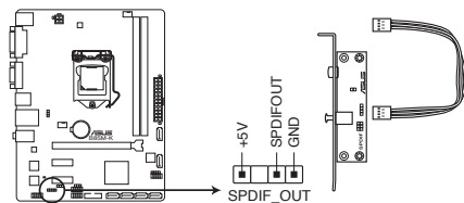
Connecteur audio numérique de la B85M-K
