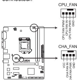
Connecteurs de ventilation de la B85M-K
