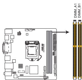
H81I-PLUS 240ピン DDR3 DIMM Slots
