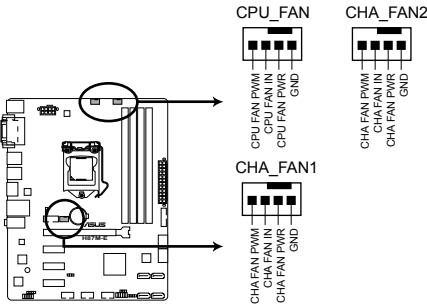
H87M-E Fan connectors
