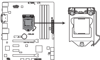
Interface de connexion LGA1150 de la H87M-PRO
