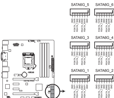
Connecteurs SATA 6.0Gbs de la H87M-PRO
