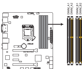
Interfaces de connexion pour modules mémoire DDR3 de la H87M-PRO
