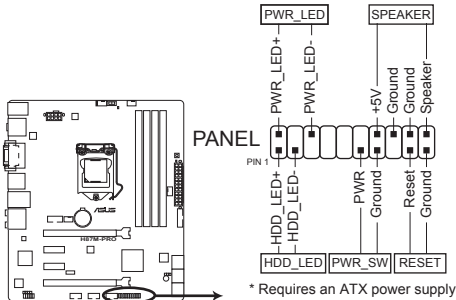
Connecteur panneau système de la H87M-PRO
