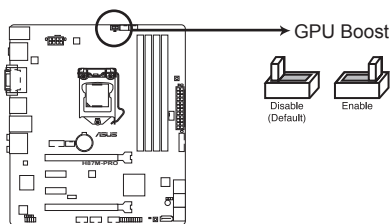
Interrupteur GPU Boost de la H87M-PRO
