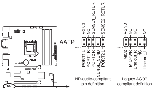
Connecteur audio pour panneau avant de la H87M-PRO
