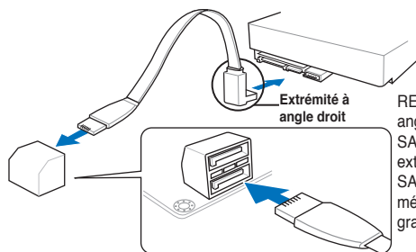
Connecteurs SATA 6.0Gbs de la H87M-PRO
