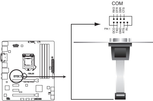
Connecteur pour port COM de la H87M-PRO
