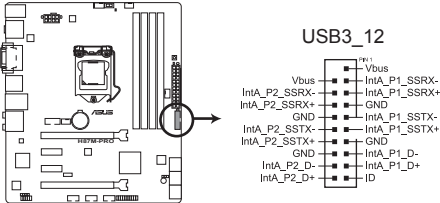
Connecteur USB 3.0 de la H87M-PRO
