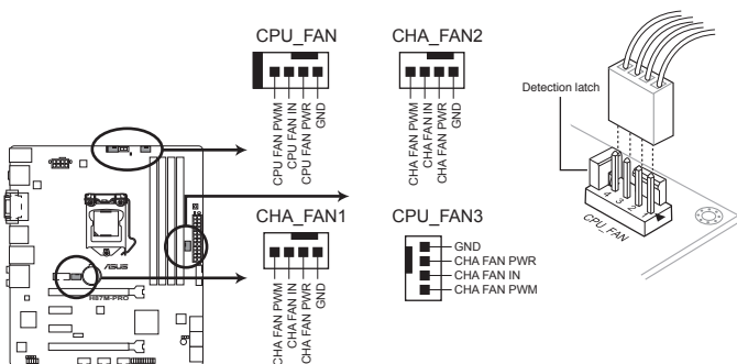
Connecteurs de ventilation de la H87M-PRO
