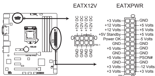
Connecteurs d'alimentation de la H87M-PRO
