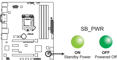
Voyant d'alimentation de la H87M-PRO
