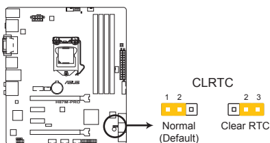
Bouton d'effacement de la mémoire CMOS de la H87M-PRO
