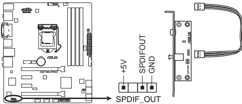
Connecteur audio numérique de la H87M-PRO
