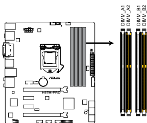
H87M-PRO 240ピンDDR3 DIMM slots
