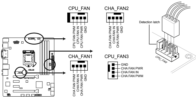
H87M-PRO Fan connectors
