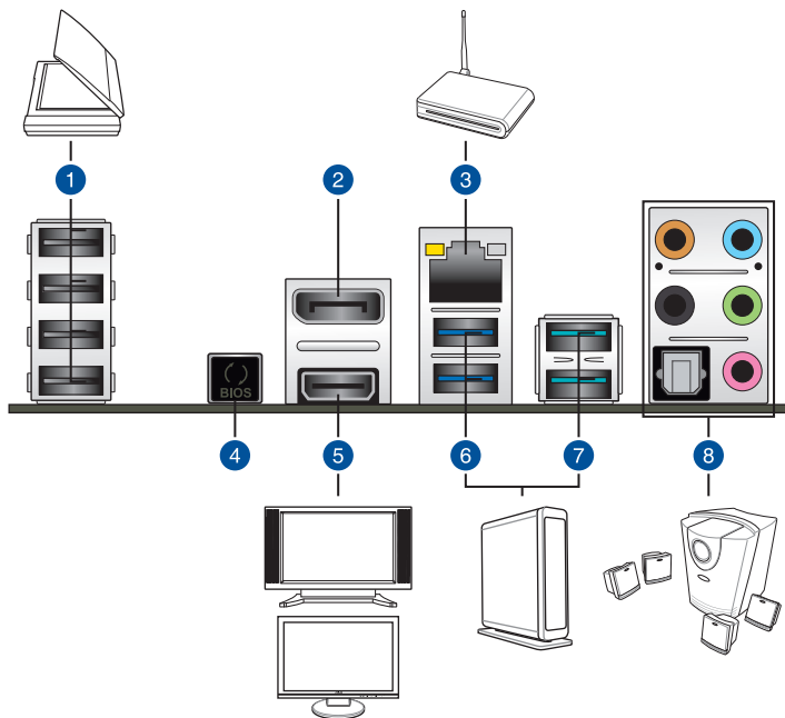
后侧面板连接埠
