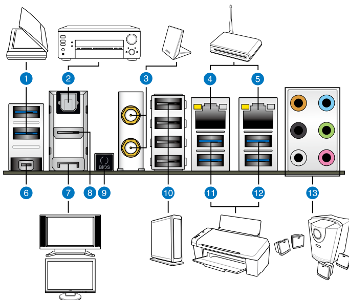
后侧面板连接端口
