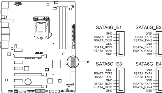
Connecteurs SATA 6Gb/s Marvell de la Z87-DELUXE
