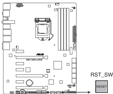
Bouton de réinitialisation de la Z87-DELUXE
