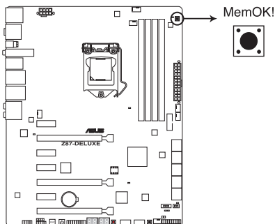
Bouton MemOK! de la Z87-DELUXE
