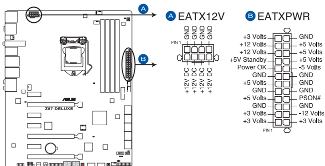
Connecteurs d'alimentation de la Z87-DELUXE
