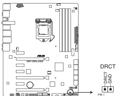
Connecteur DirectKey de la Z87-DELUXE
