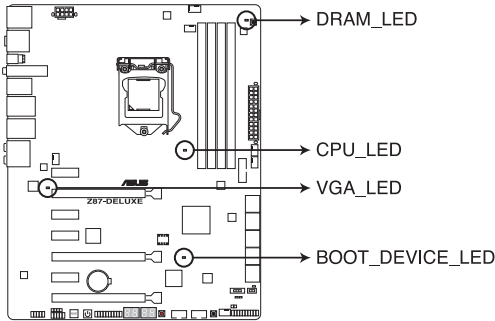
LED du POST de la Z87-DELUXE
