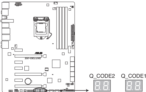
LED de débogage de la Z87-DELUXE
