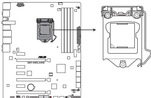
Interface de connexion LGA1150 de la Z87-DELUXE
