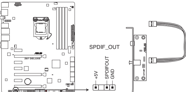
Connecteur audio numérique de la Z87-DELUXE
