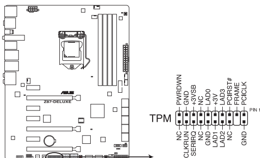
Connecteur TPM de la Z87-DELUXE
