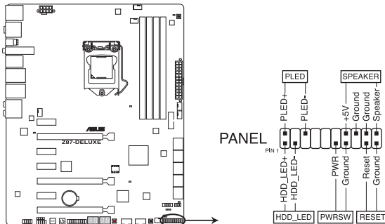
Connecteur panneau système de la Z87-DELUXE
