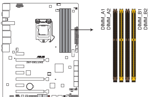
Interfaces de connexion pour modules mémoire DDR3 de la Z87-DELUXE
