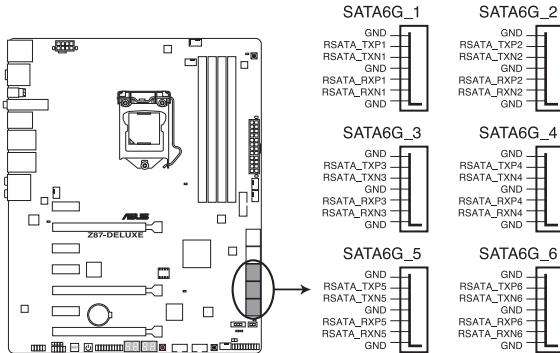
Connecteurs SATA 6.0Gbs de la Z87-DELUXE
