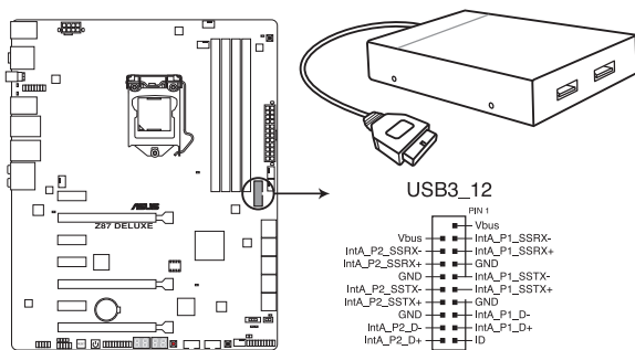
Connecteur USB 3.0 de la Z87-DELUXE
