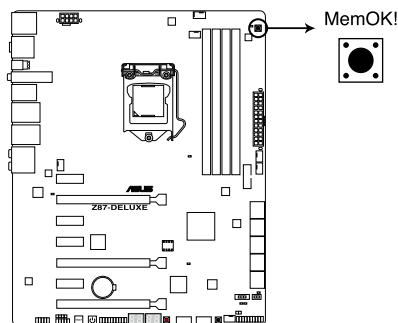
Z87-DELUXE MemOK! button
