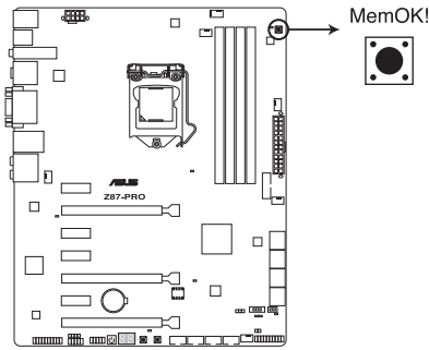
Z87-PRO MemOK! button
