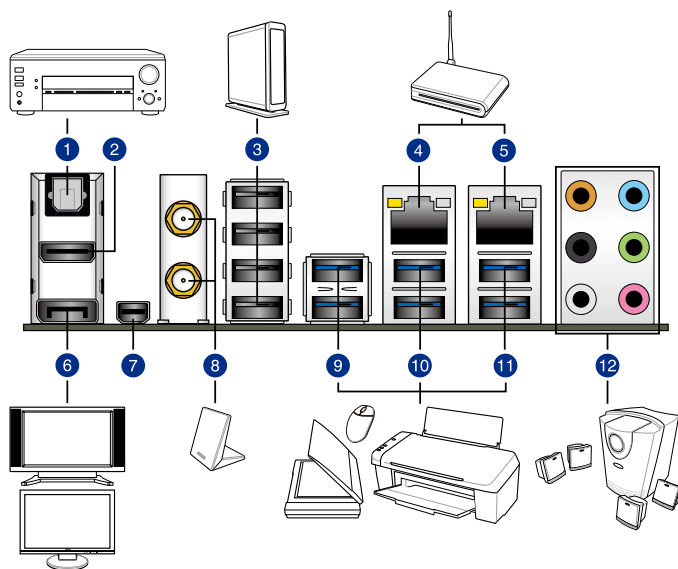
后侧面板连接端口
