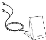
1 x 2T2R 双频 Wi-Fi 移动天线 (与 Wi-Fi 802.11a/b/g/n/ac 兼容)
