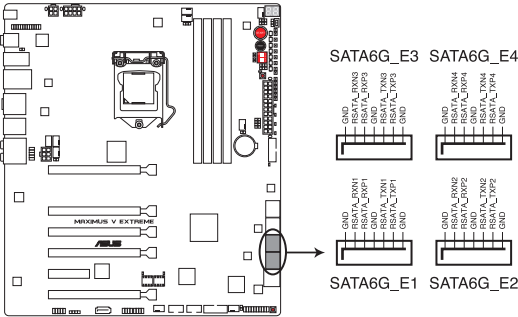
Connecteurs SATA 6Gb/s Marvell de la MAXIMUS V EXTREME
