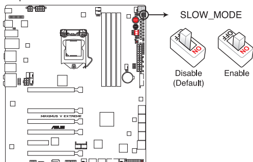
Interrupteur Slow Mode de la MAXIMUS V EXTREME
