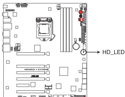
LED d'activité de disque dur de la MAXIMUS V EXTREME
