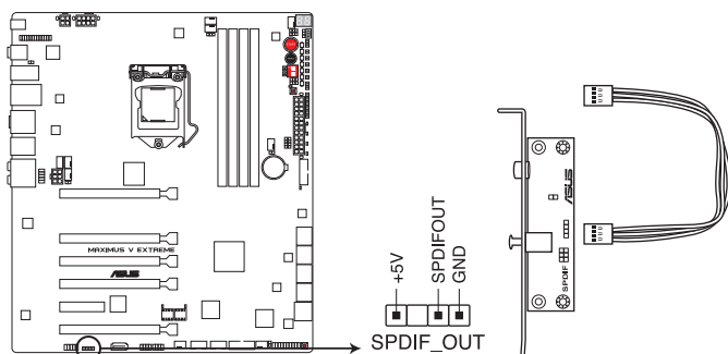
Connecteur audio numérique de la MAXIMUS V EXTREME
