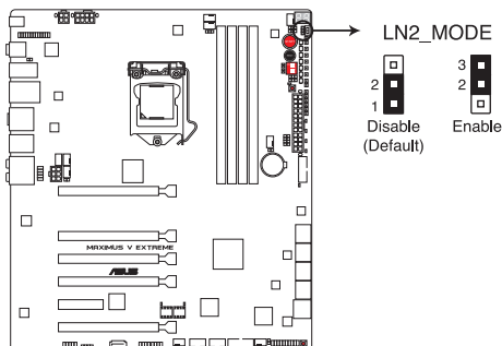
Jumper LN2 de la MAXIMUS V EXTREME
