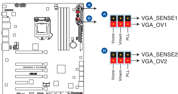
Connecteur VGA Hotwire de la MAXIMUS V EXTREME
