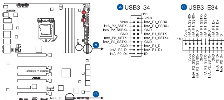
Connecteurs USB 3.0 de la MAXIMUS V EXTREME
