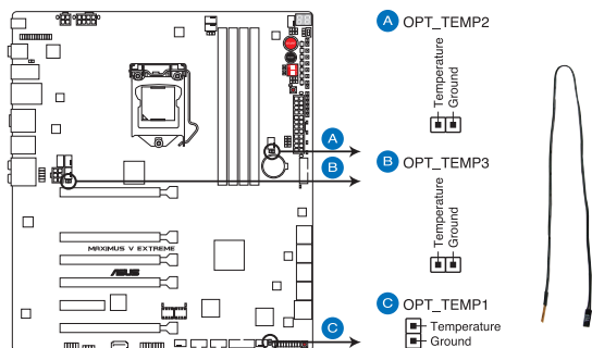
Connecteurs pour capteurs thermique de la MAXIMUS V EXTREME
