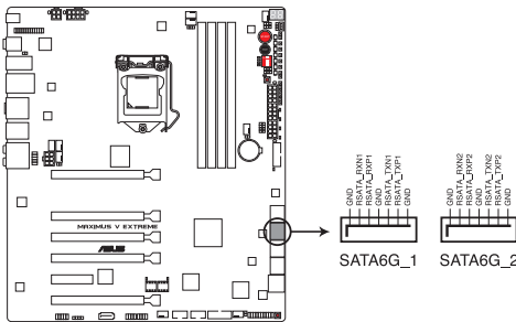
Connecteurs SATA 6.0Gbs de la MAXIMUS V EXTREME
