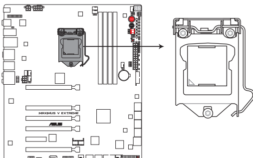
Interface de connexion LGA1155 de la MAXIMUS V EXTREME
