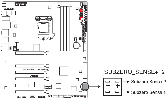
Connecteur Subzero Sense de la MAXIMUS V EXTREME
