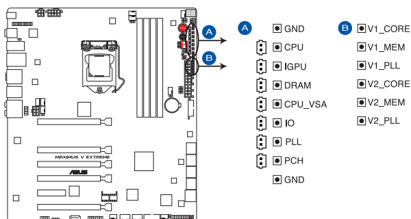
Zone Probelt de la MAXIMUS V EXTREME
