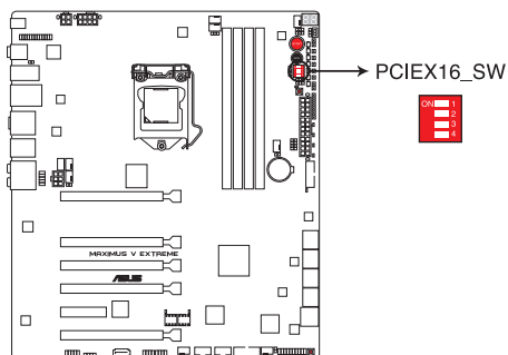
Interrupteurs de voie PCIe x16 de la MAXIMUS V EXTREME
