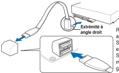
Connecteurs SATA 6.0Gbs de la MAXIMUS V EXTREME
