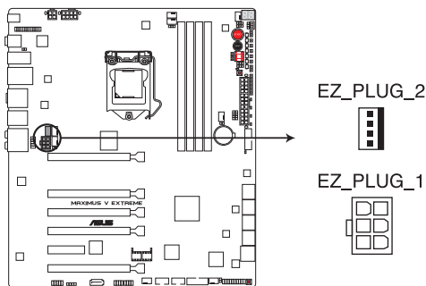
Connecteurs EZ Plug de la MAXIMUS V EXTREME
