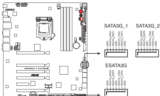
Connecteurs SATA 3Gb/s de la MAXIMUS V EXTREME
