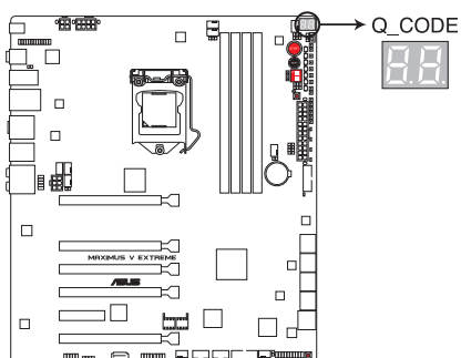
LED de débogage de la MAXIMUS V EXTREME
