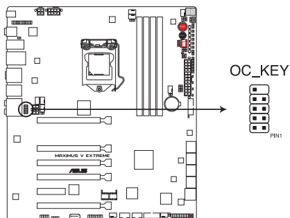
Connecteur OC Key de la MAXIMUS V EXTREME
