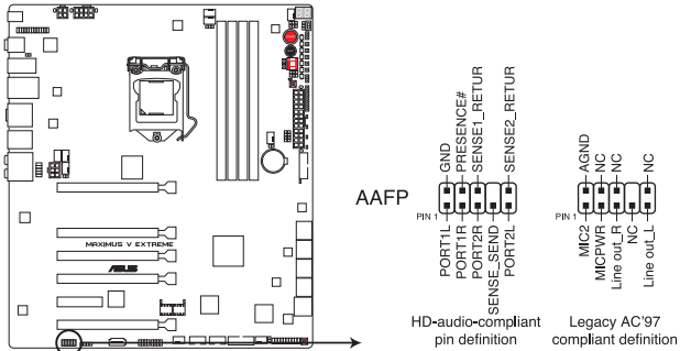
Connecteur audio pour panneau avant de la MAXIMUS V EXTREME
