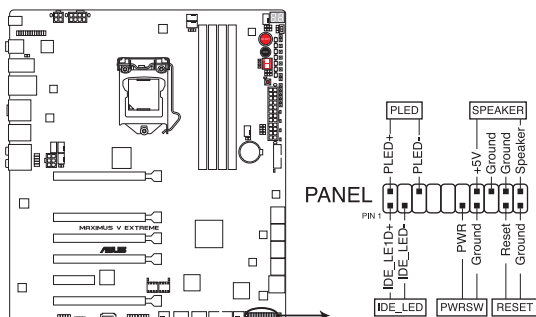
Connecteur panneau système de la MAXIMUS V EXTREME
