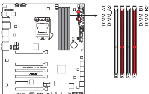
Interfaces de connexion pour modules mémoire DDR3 de la MAXIMUS V EXTREME
