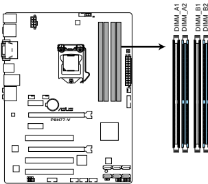
Slots DDR3 de la P8H77-V
