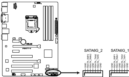
Connecteurs SATA 6.0Gbs de la P8H77-V
