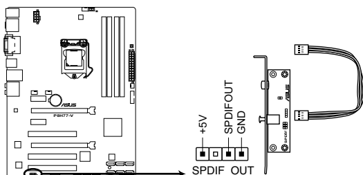
Connecteur audio numérique de la P8H77-V
