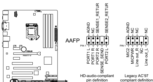
Connecteur audio pour panneau avant de la P8H77-V
