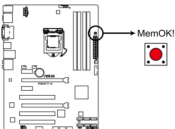
Interrupteur MemOK! de la P8H77-V
