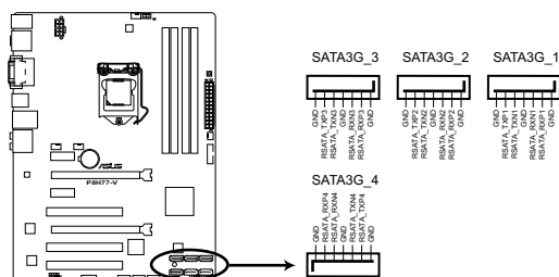
Connecteurs SATA 3Gb/s de la P8H77-V
