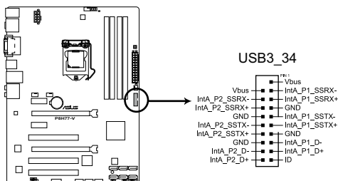
Connecteur USB 3.0 de la P8H77-V
