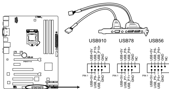
Connecteurs USB 2.0 de la P8H77-V
