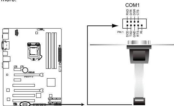
Connecteur COM de la P8H77-V
