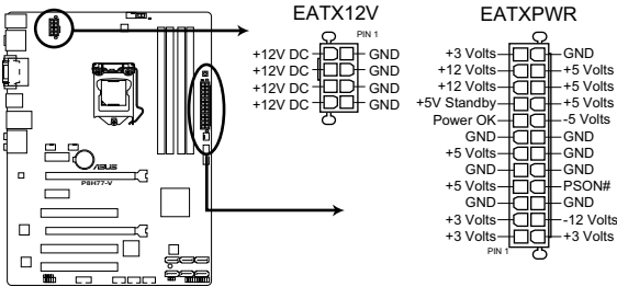
Connecteurs d'alimentation de la P8H77-V
