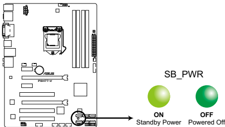
LED d'alimentation de la P8H77-V
