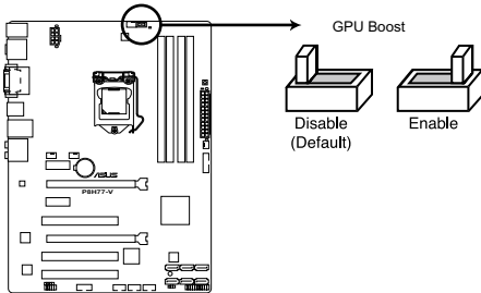
Interrupteur GPU Boost de la P8H77-V
