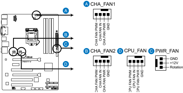
Connecteurs de ventilation de la P8H77-V
