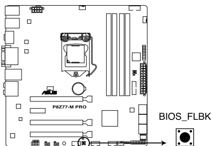
Bouton USB BIOS Flashback de la P8Z77-M PRO
