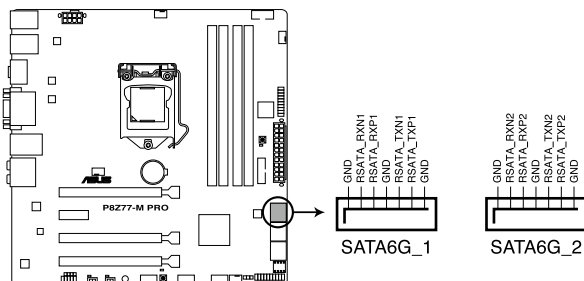
Connecteurs SATA 6.0Gbs de la P8Z77-M PRO
