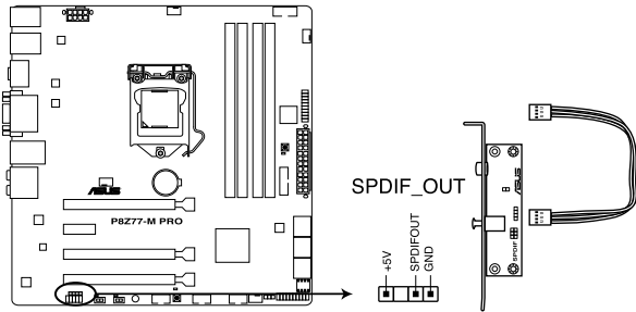
Connecteur audio numérique de la P8Z77-M PRO
