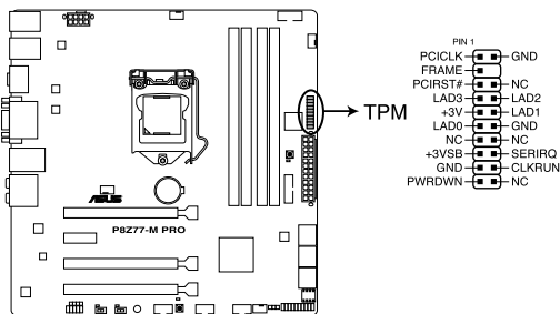
Connecteur TPM de la P8Z77-M PRO
