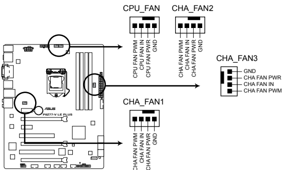
P8277-V LE PLUS fan connectors
