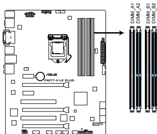
P8Z77-V LE PLUS 240-pin DDR3 DIMM sockets
