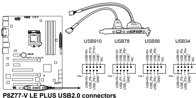
P8277-V LE PLUS USB2.0 connectors
