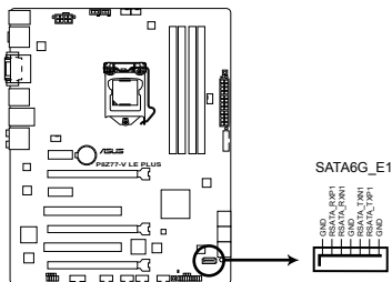
P8Z77-V LE PLUS Marvell® SATA 6.0 Gb/s connector
