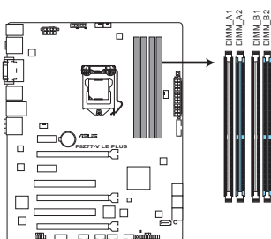
Slots DDR3 de la P8Z77-V LE PLUS
