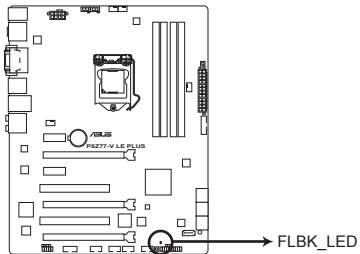
LED BIOS Flashback de la P8Z77-V LE PLUS
