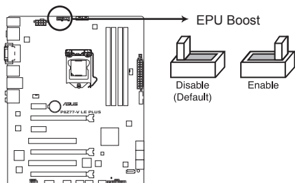
Interrupteur EPU de la P8Z77-V LE PLUS
