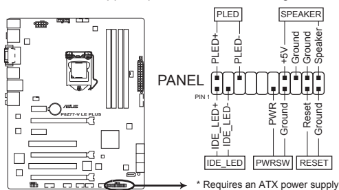
Connecteur panneau système de la P8Z77-V LE PLUS
