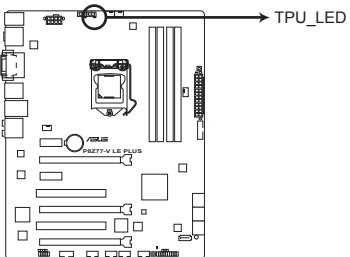
LED EPU de la P8Z77-V LE PLUS
