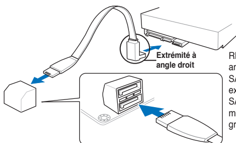
Connecteurs SATA 6.0Gbs de la P8Z77-V LE PLUS
