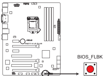
Bouton BIOS Flashback de la P8Z77-V LE PLUS
