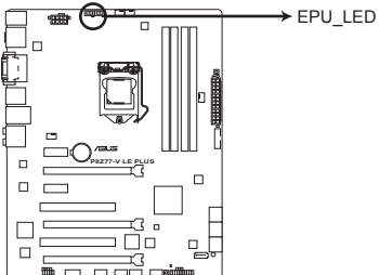
LED TPU de la P8Z77-V LE PLUS
