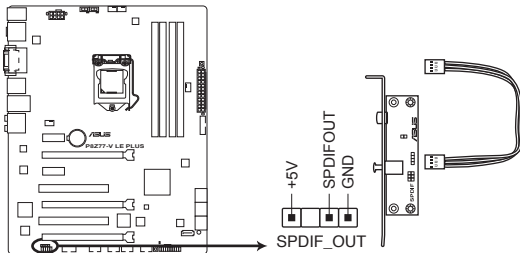
Connecteur audio numérique de la P8Z77-V LE PLUS
