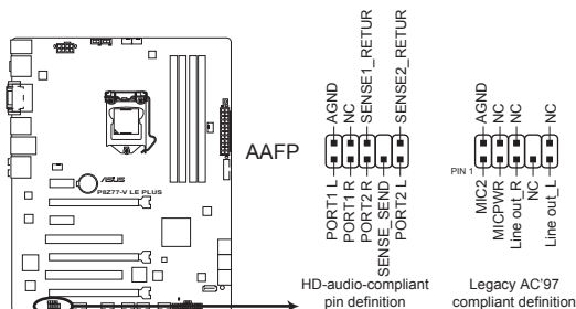
Connecteur audio pour panneau avant de la P8Z77-V LE PLUS
