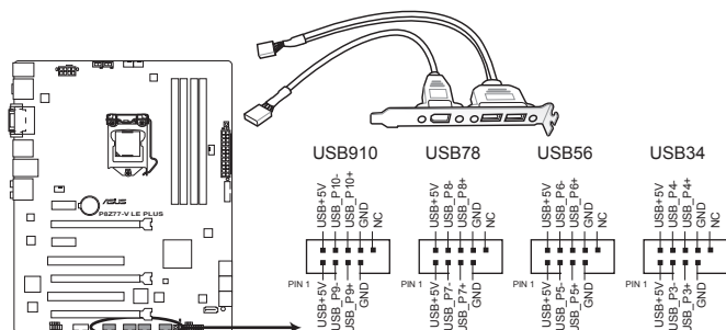
Connecteurs USB 2.0 de la P8Z77-V LE PLUS
