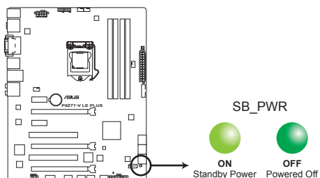
LED d'alimentation de la P8Z77-V LE PLUS
