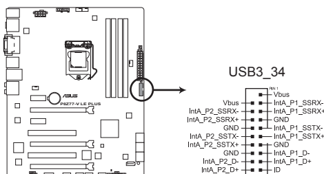
Connecteur USB 3.0 de la P8Z77-V LE PLUS
