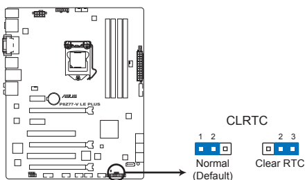
Jumper d'effacement de la mémoire CMOS de la P8Z77-V LE PLUS
