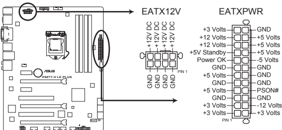
Connecteurs d'alimentation de la P8277-V LE PLUS
