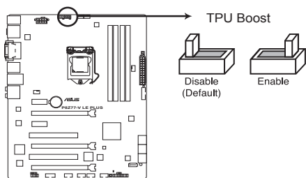
Interrupteur TPU de la P8Z77-V LE PLUS
