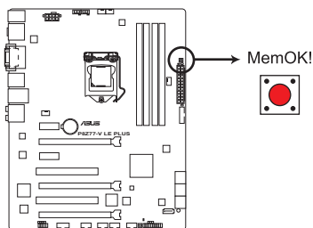
Interrupteur MemOK! de la P8Z77-V LE PLUS
