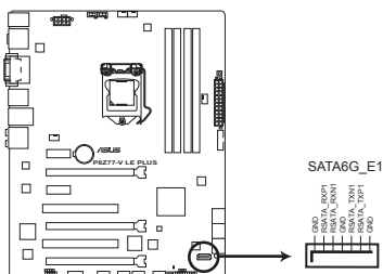
Connecteur SATA 6Gb/s Marvell de la P8277-V LE PLUS
