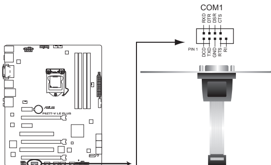
Connecteur pour port COM de la P8Z77-V LE PLUS
