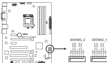
Connecteurs SATA 6.0Gbs de la P8Z77-V LE PLUS
