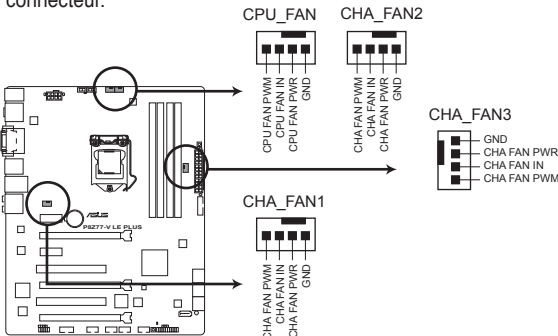
Connecteurs de ventilation de la P8Z77-V LE PLUS
