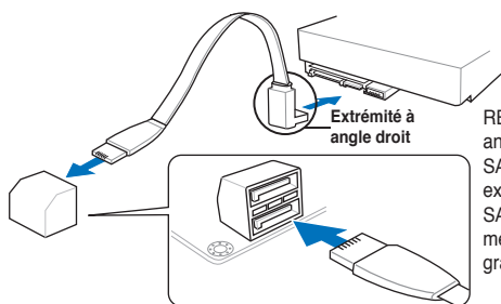
Connecteurs SATA 3Gb/s de la P8Z77-V LE PLUS
