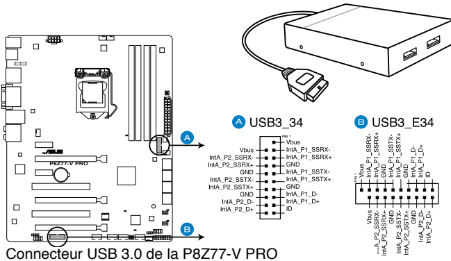
Connecteur USB 3.0 de la P8Z77-V PRO
