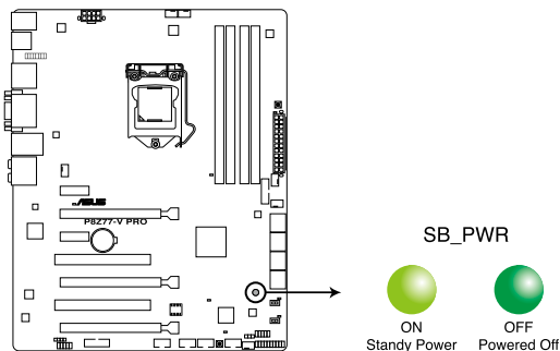
LED d'alimentation de la P8Z77-V PRO
