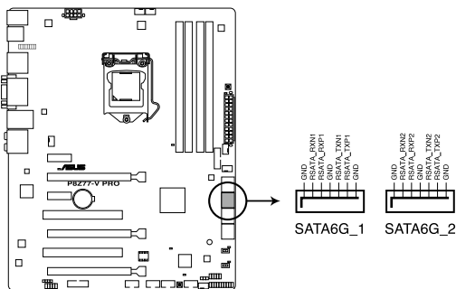
Connecteurs SATA 6.0Gbs de la P8Z77-V PRO
