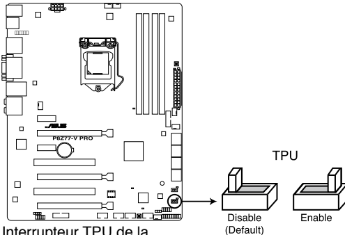
Interrupteur TPU de la P8Z77-V PRO
