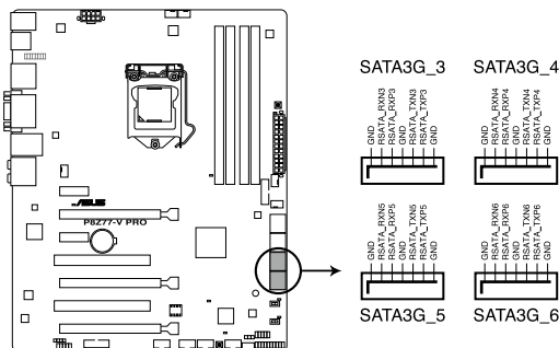
Connecteurs SATA 3Gb/s de la P8Z77-V PRO
