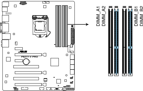
Slots DDR3 de la P8Z77-V PRO
