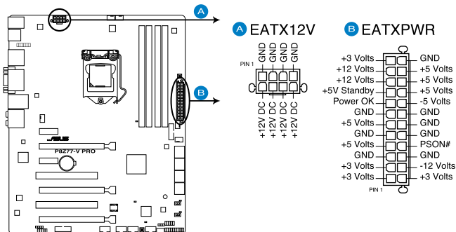
Connecteurs d'alimentation de la P8Z77-V PRO
