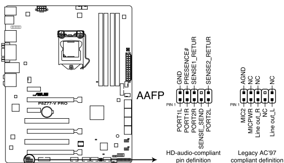
Connecteur audio pour panneau avant de la P8Z77-V PRO
