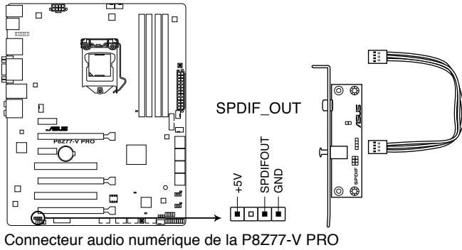
Connecteur audio numérique de la P8Z77-V PRO
