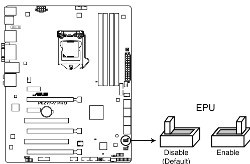
Interrupteur EPU de la P8Z77-V PRO
