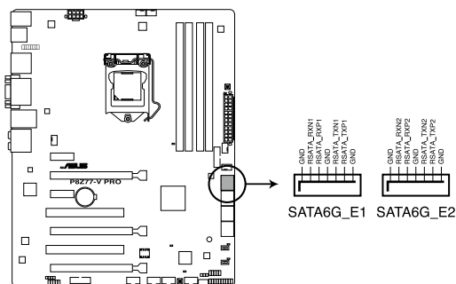
Connecteur SATA 6Gb/s Marvell de la P8Z77-V PRO
