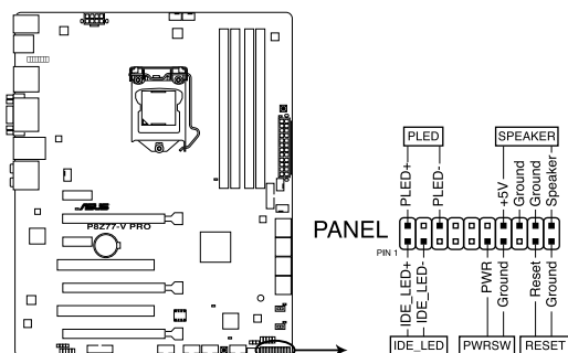
Connecteur panneau système de la P8Z77-V PRO
