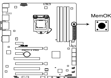
Interrupteur MemOK! de la P8Z77-V PRO
