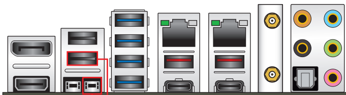
BIOS FlashBack™ ボタン BIOS FlashBack™ ポート
