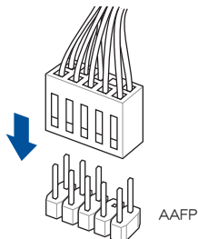
安装前面板音频接针
