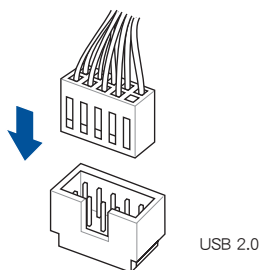
安装 USB 2.0 接针
