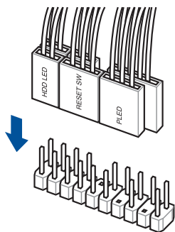
安装系统控制面板接针
