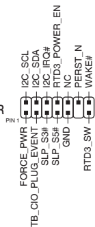
TB(USB4)_HEADER
