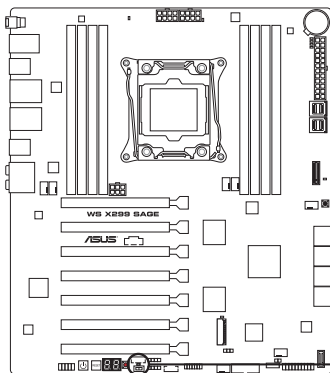
WS X299 SAGE XLED1
