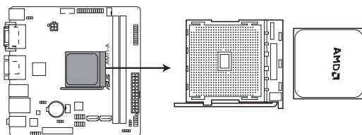
Socket de l'APU de la AM1-A
