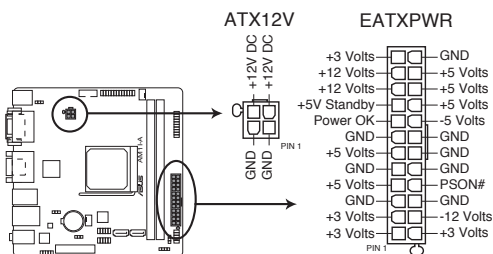
Connecteurs ATX de la AM11-A
