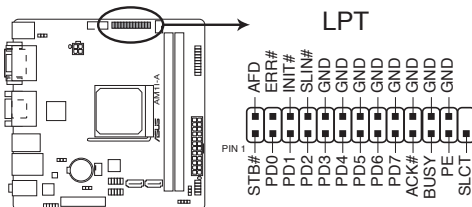
Connecteur LPT de la AM11-A
