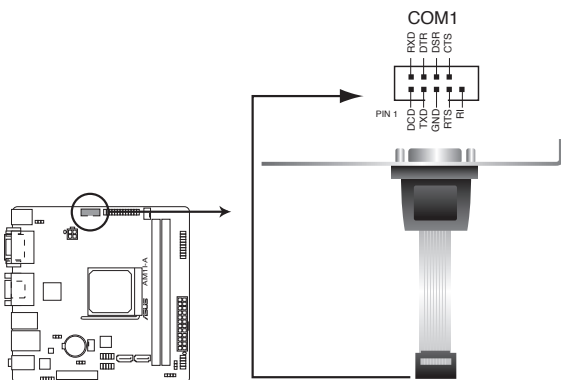
Connecteur pour port COM de la AM11-A
