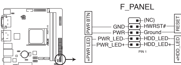
Connecteur système de la AM11-A
