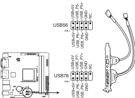
Connecteurs USB 2.0/1.1 de la AM11-A
