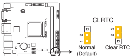
Jumper d'effacement de la mémoire RTC de la AM11-A
