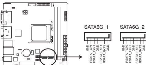
Connecteurs SATA de la AM11-A
