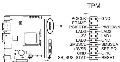
Connecteur TPM de la A85M-E
