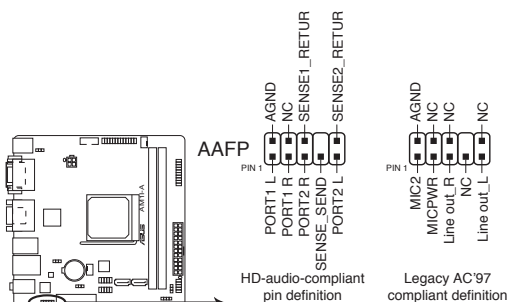
Connecteur pour port audio en façade de la AM11-A
