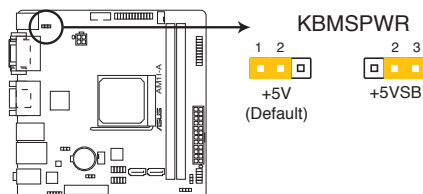
Jumper de mise en route via clavier/souris de la AM11-A
