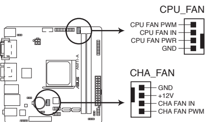
Connecteurs de ventilation de la AM11-A
