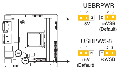
Jumper de mise en route via USB de la AM11-A
