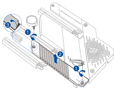
M.2_2 (類型 22110 M.2)
