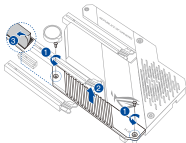
M.2_2 (類型 2242 / 2260 / 2280 M.2)
