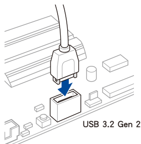
安裝 USB 3.2 Gen 2 連接插槽
