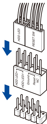
安裝 ASUS Q-Connector
