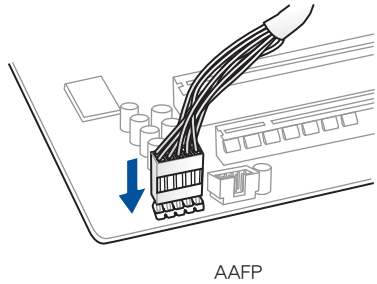
安装前面板音频连接插槽
