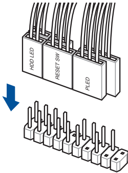
安装前面板连接插槽
