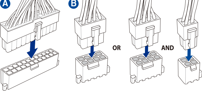
تنصيب توصيلات الطاقة ATX رابط های برق ATX را نصب کنید
