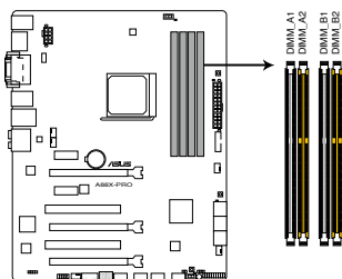
A88X-PRO 240ピン DDR3 DIMM Slots
