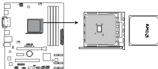
A88XM-A CPU socket FM2+
