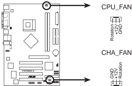
P4P800S-X 12-Volt Fan Connectors
