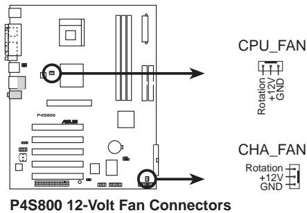
P4S800 12-Volt Fan Connectors
