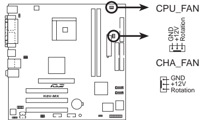
K8V-MX Fan connectors
