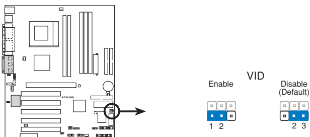
A7A266 VID Selection
