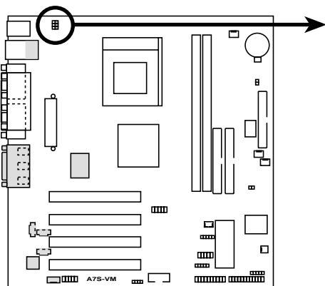
A7S-VM USB Wake Up
