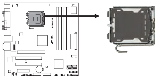
Socket 775 de la P5B-VM
