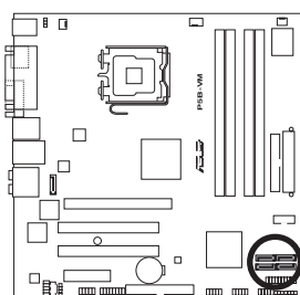
Connecteurs SATA de la P5B-VM
