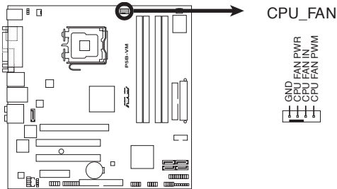
Connecteur CPU_FAN de la P5B-VM
