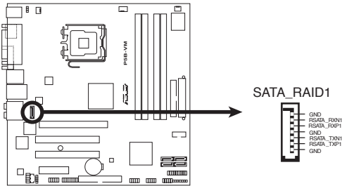
Connecteur RAID SATA de la P5B-VM
