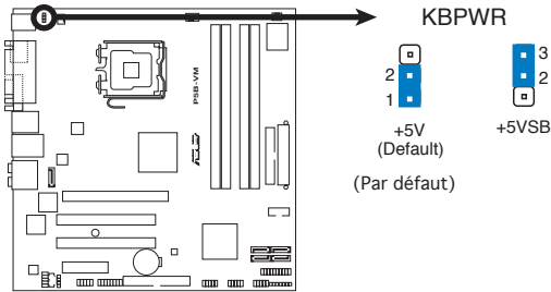
Paramètres d'alimentation du clavier de la P5B-VM
