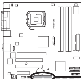
Connecteur IDE de la P5B-VM
