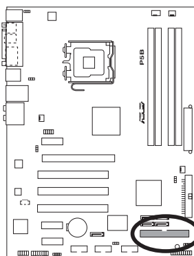
P5B IDE-Anschluss
