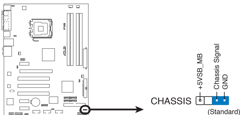
P5B Gehäuseeinbruchsanschluss
