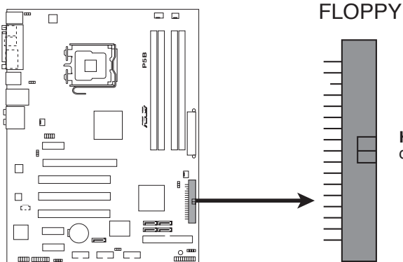
P5B Diskettenlaufwerksanschluss
