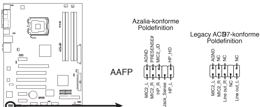
P5B Fronttafelaudioanschluss
