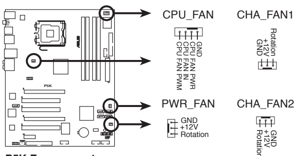
P5K Fan connectors
