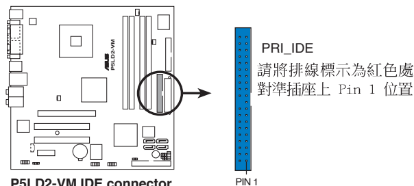
P5LD2-VM IDE connector
