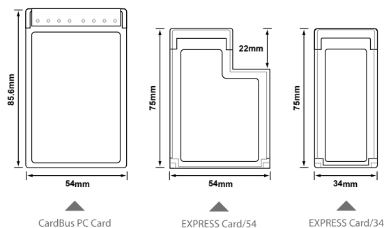
▲CardBus PC卡跟EXPRESSCard/34、EXPRESSCard/54的比較
