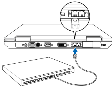
區域網路連接
