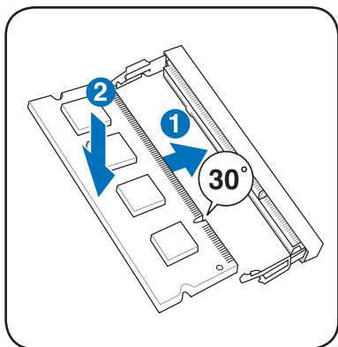
安装内存条
