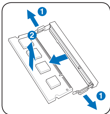
移除内存条
